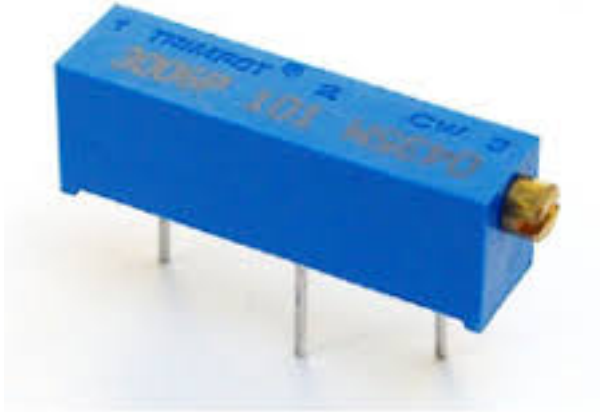
Cermet-Potentiometer
