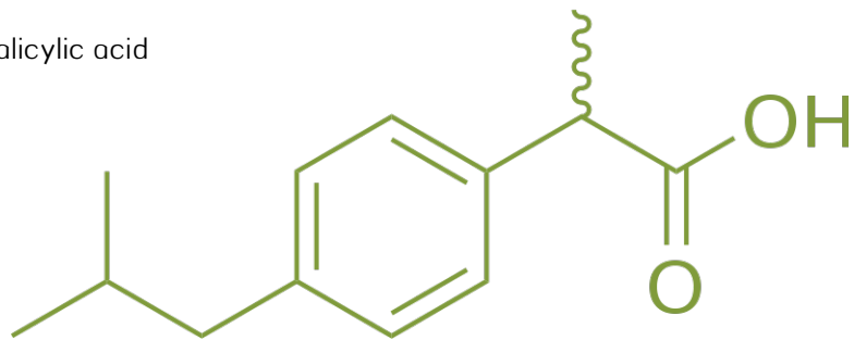
Ibuprofen
